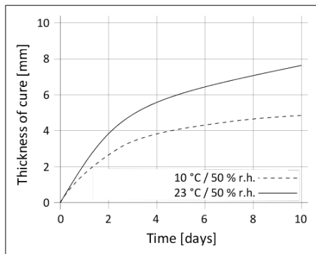
Diagram 1: Rychlost vytvrzování Sikaflex®-522
