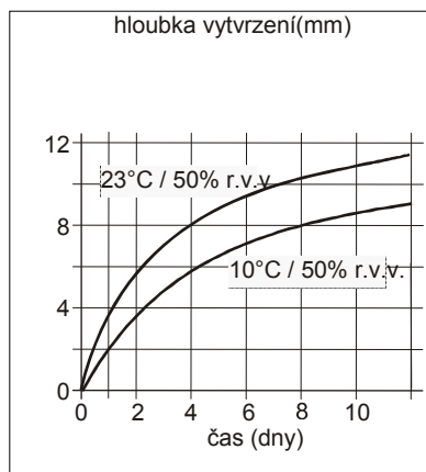
Diagram 1: rychlost vytvrzování pro SikaTack Go4it!
