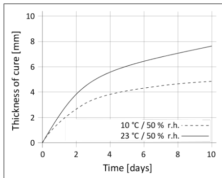
Diagram 1: Rychlost vytvrzování Sikaflex®-521 UV
