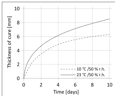
Diagram 1: Rychlost vytvrzení Sikaflex®-552 AT
