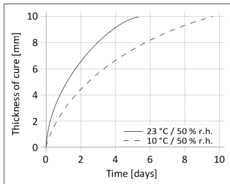
Graf 1: Rychlost vytvrzování Sikaflex®-221 LV
