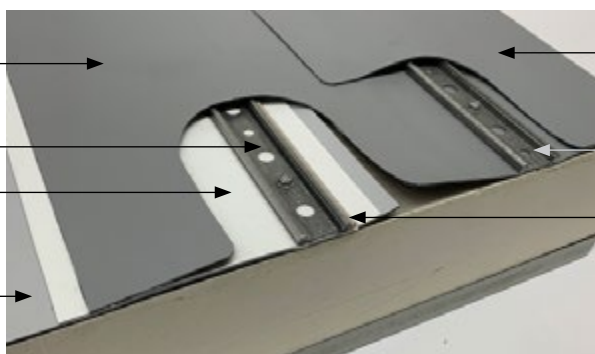
4. Automatické horkovzdušné navaření FPO Sarnafil® fólie na pásku SikaRoof® Multitape.
