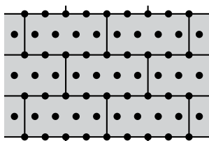
Rozmístění hmoždinek při počtu 14 ks na m²
