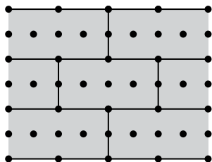
Rozmístění hmoždinek při počtu 8,3 ks na m²
