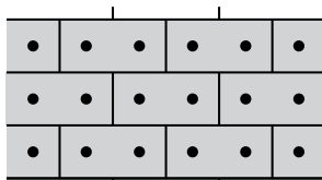
Rozmístění hmoždinek při počtu 6 ks na m 2
