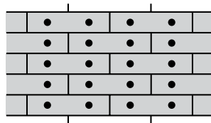
Rozmístění hmoždinek při počtu 10 ks na m²
