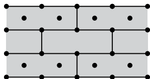
Rozmístění hmoždinek při počtu 6,5 ks na m²
