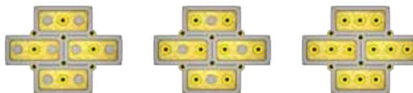
Kotvení a lepicí plán izolačních desek 1000 × 600 mm
