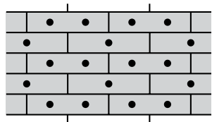
Rozmístění hmoždinek při počtu 8 ks na m²
