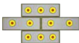
Rozmístění hmoždinek a lepidla při počtu 8 ks na m 2
