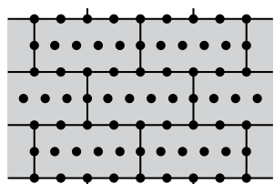
Rozmístění hmoždinek při počtu 16 ks na m²
