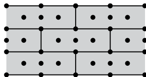
Rozmístění hmoždinek při počtu 10 ks na m²
