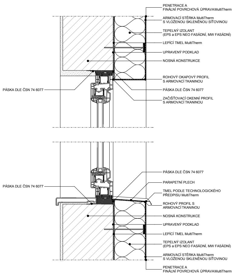
Podélný řez parapetem - A
