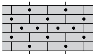
Rozmístění hmoždinek při počtu 6 ks na m²
