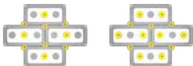
Kotvení a lepicí plán izolačních desek 1000 × 500 mm
