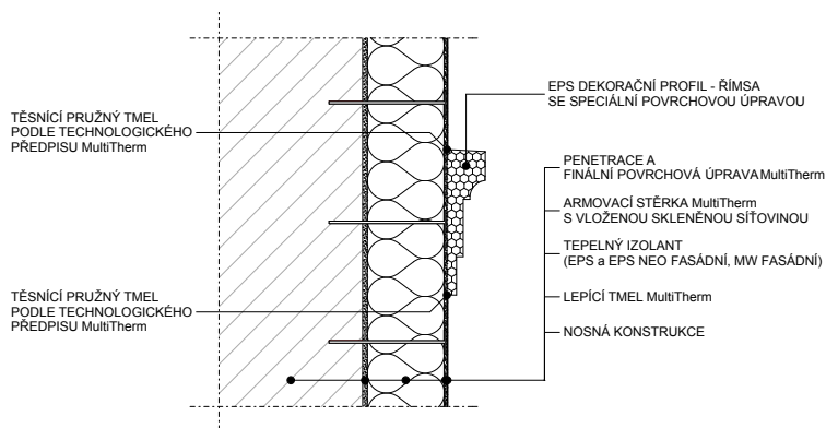
Římsa z dekoračního profilu
