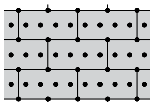
Rozmístění hmoždinek při počtu 10 ks na m²
