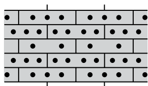
Rozmístění hmoždinek při počtu 16 ks na m²
