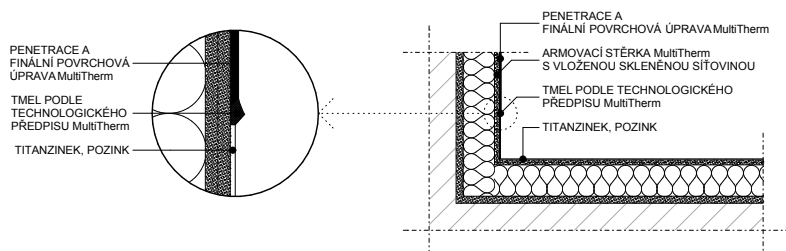
Podélný řez parapetem - zapuštěný profil
