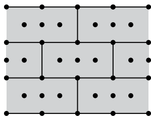
Rozmístění hmoždinek při počtu 6,5 ks na m²
