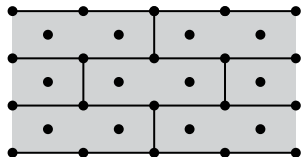
Rozmístění hmoždinek při počtu 8,8 ks na m²
