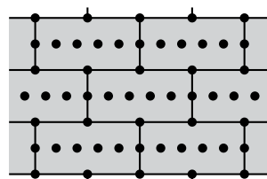
Rozmístění hmoždinek při počtu 12 ks na m²
