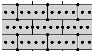
Rozmístění hmoždinek při počtu 16 ks na m 2
