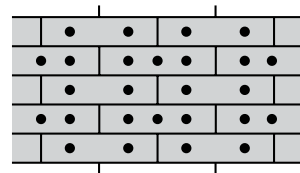
Rozmístění hmoždinek při počtu 12 ks na m²
