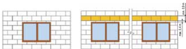
Řešení bez protipožárního pásu z MW se schválením PKO
