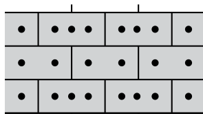
Rozmístění hmoždinek při počtu 8 ks na m 2
