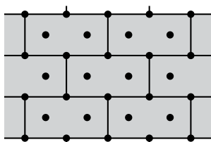
Rozmístění hmoždinek při počtu 6 ks na m²
