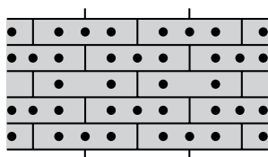
Rozmístění hmoždinek při počtu 14 ks na m²
