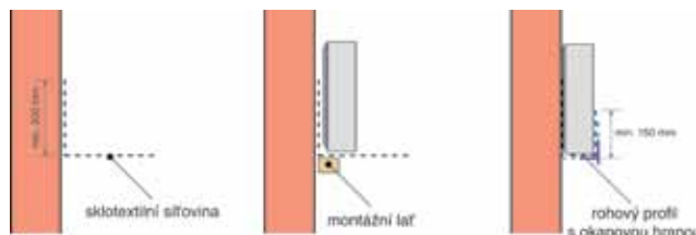
Založení systému s pomocí montážní latě
