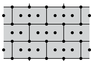
Rozmístění hmoždinek při počtu 8 ks na m²
