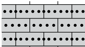
Rozmístění hmoždinek při počtu 14 ks na m 2
