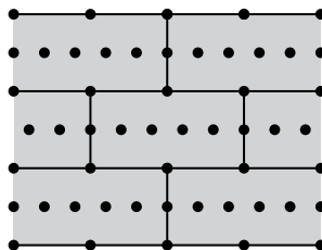
Rozmístění hmoždinek při počtu 10,8 ks na m²
