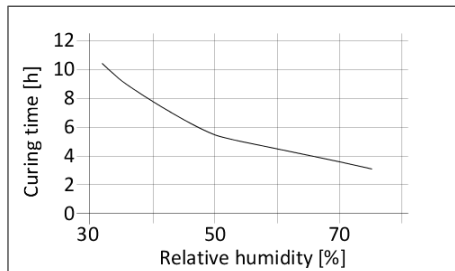
Diagram 1: Doba vytvrzení pro tloušťku filmu 500 µm
