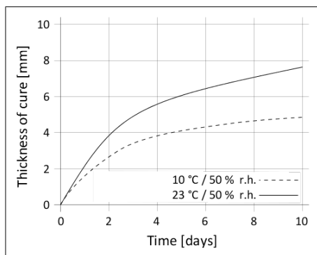
Diagram 1: Rychlost vytvrzování Sikaflex®-521 UV
